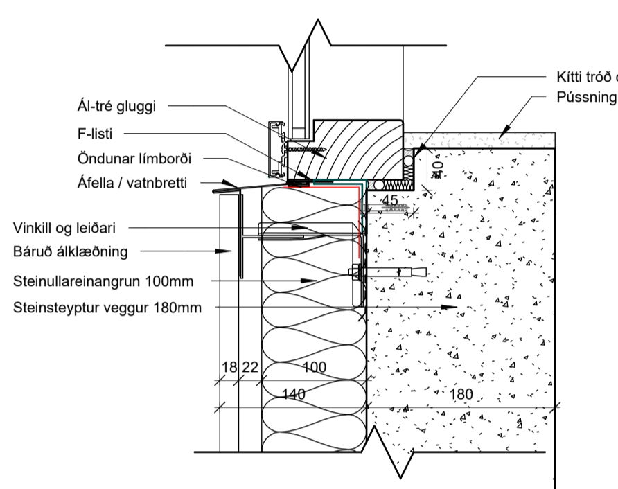
2 Undir glugga báruál 1 : 5
