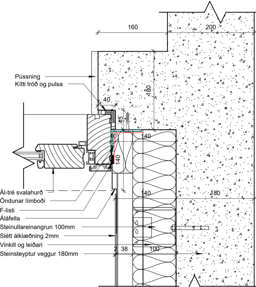
4 Innhorn slétt ál að svalahurð 1 : 5
