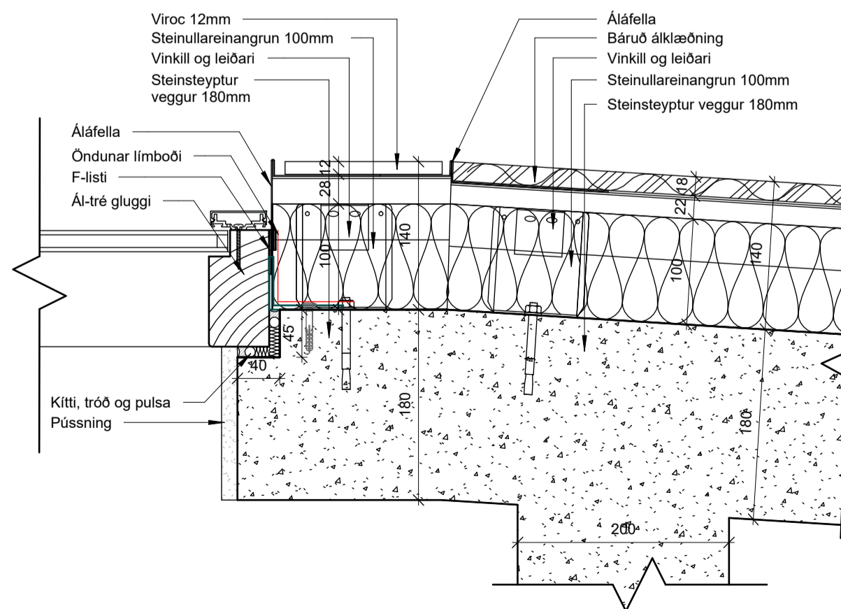
8 Úthorn gleitt báru að Viroc 1 : 5
