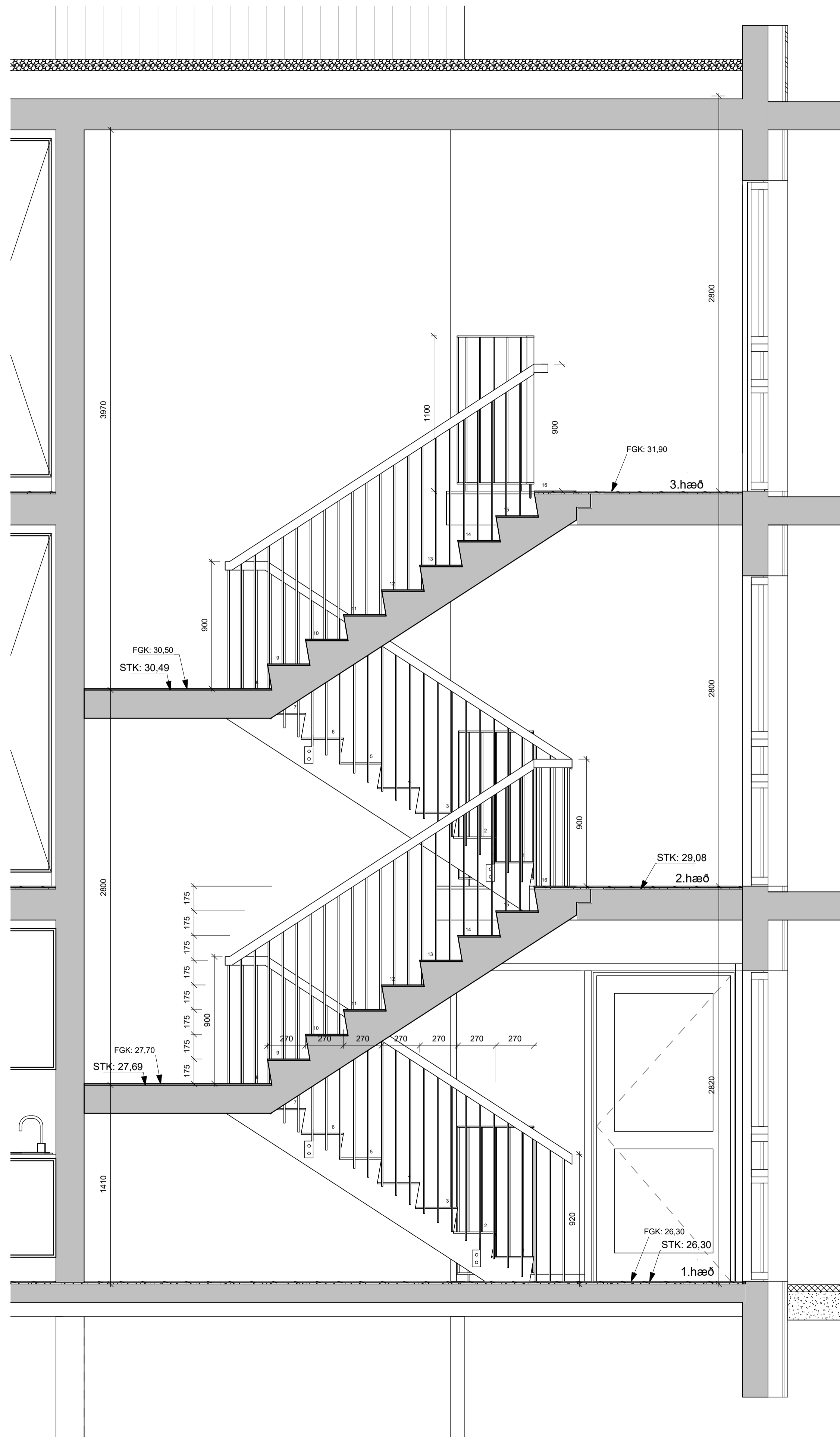
2 Snið 1 : 20
