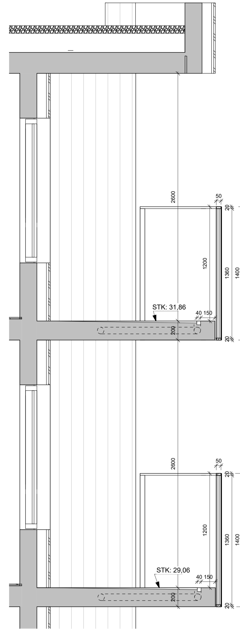
2 Snið í svalir 0205- 0206- 0306- 0307 1 : 20
