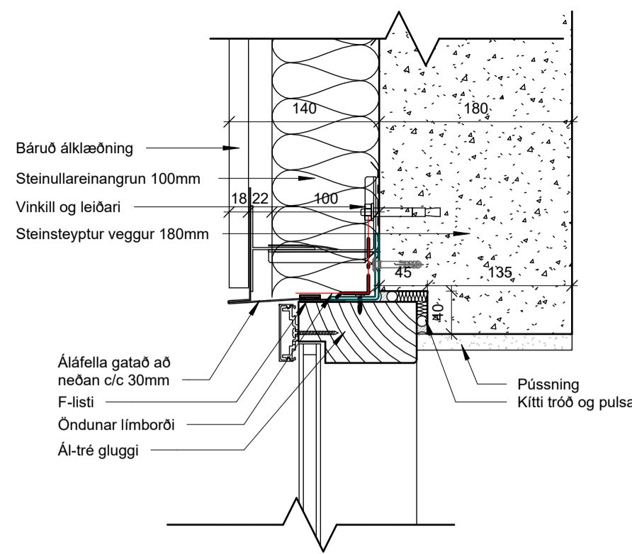
1 Yfir glugga báruál 1 : 5
