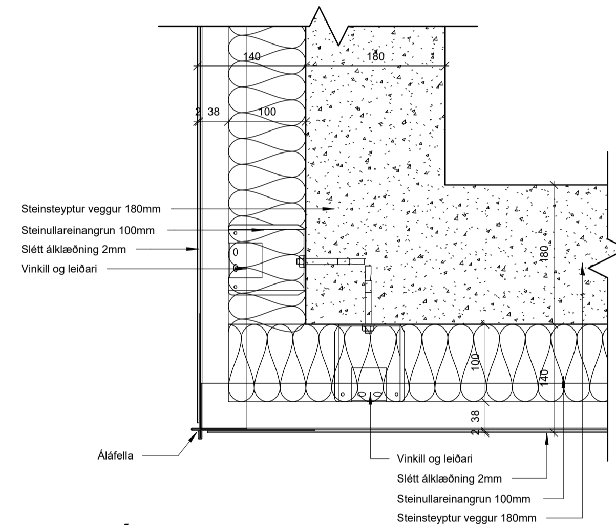
9 Úthorn slétt ál 1 : 5
