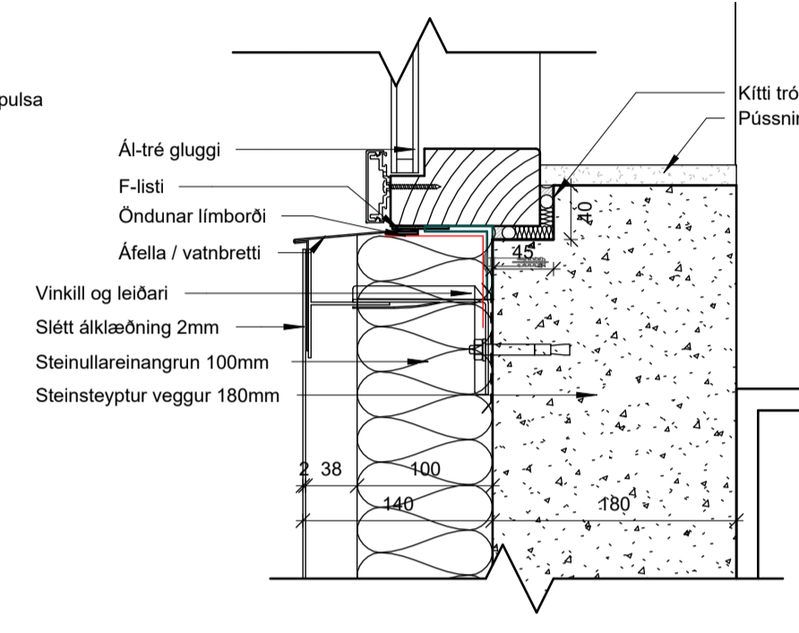
6 Undir glugga slétt ál 1 : 5
