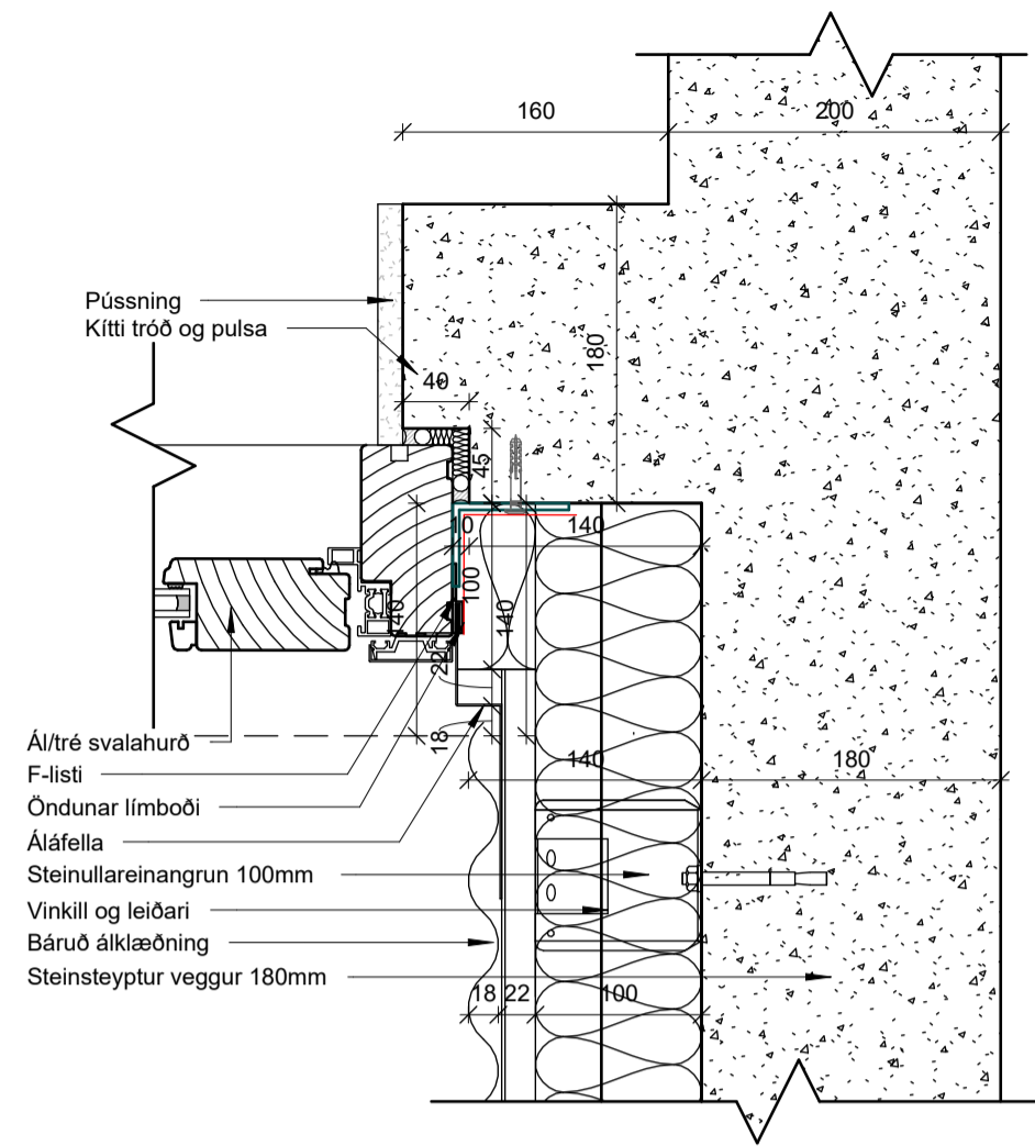
1 Innhorn báruál með hurð 1 : 5
