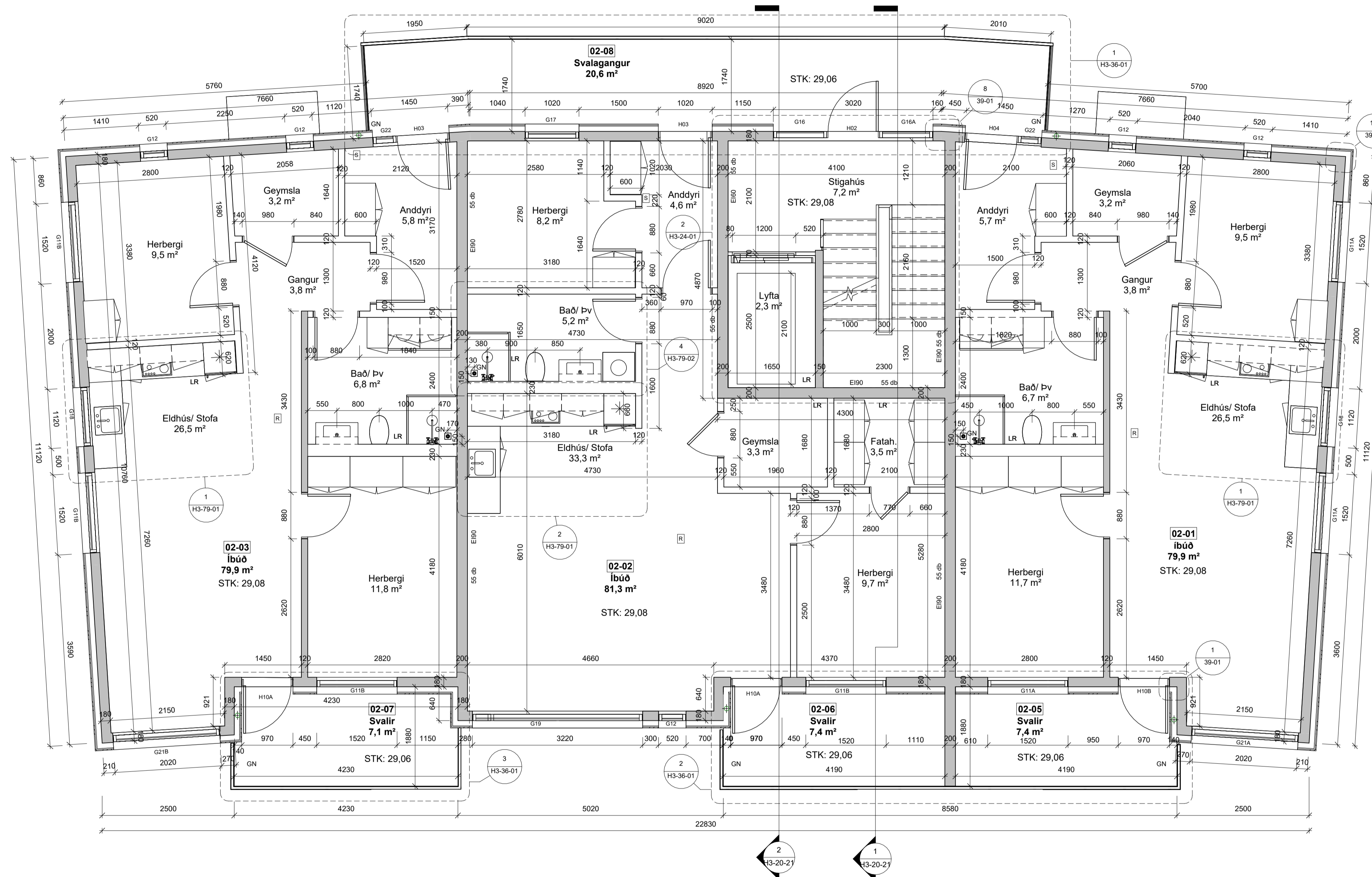
1 2. hæð 1:50
