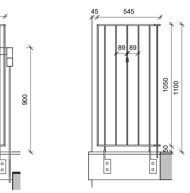
6 Handrið við lyftu 3. hæð 1:20
