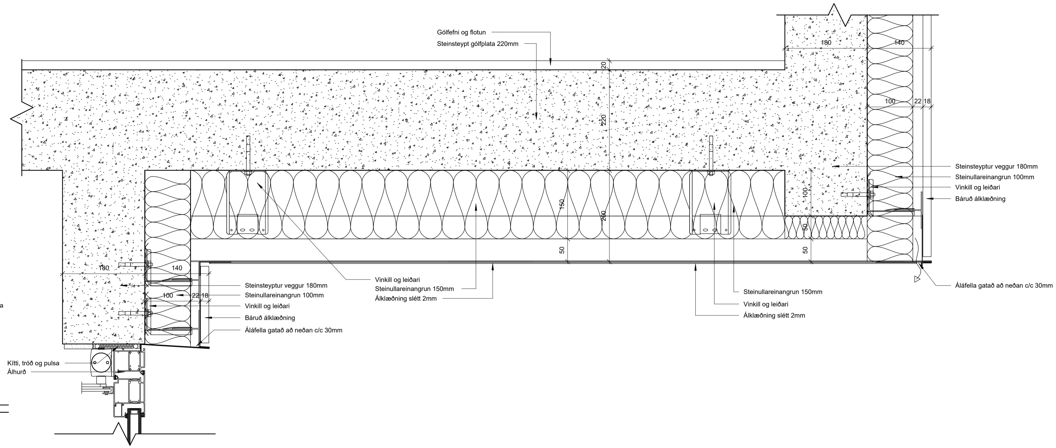
3 Yfir anddyri 1 : 5
