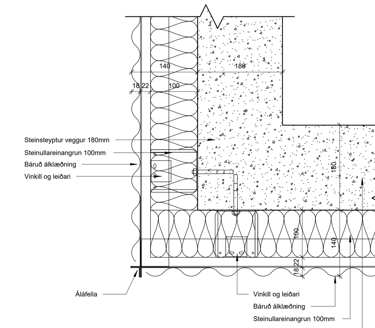
11 Úthorn báruál 1 : 5
