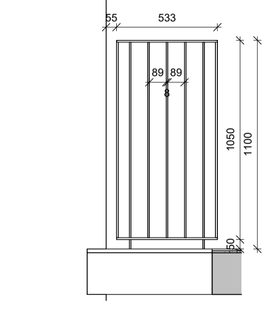
7 Handrið við lyftu 1.-2. hæð 1:20
