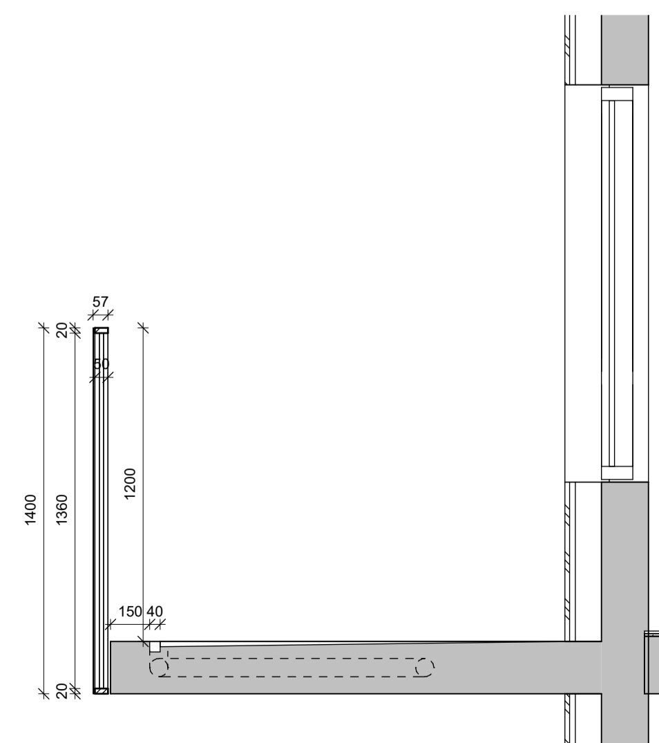
4 Snið í svalir 0207-0308 1 : 20
