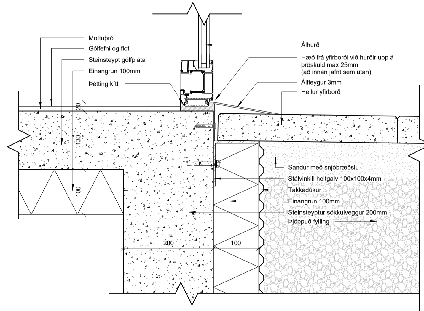
9 Hurð í anddyri 1 : 5
