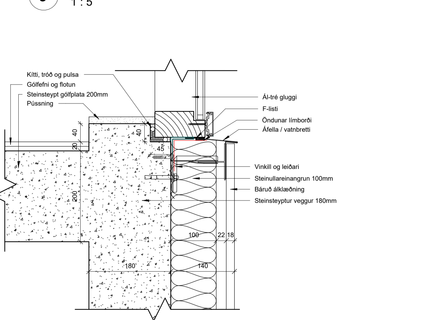
4 Undir gólfsiðan glugga bára 1 : 5
