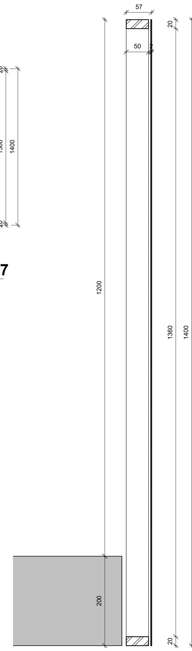
6 Snið í svalahandrið 1 : 5
