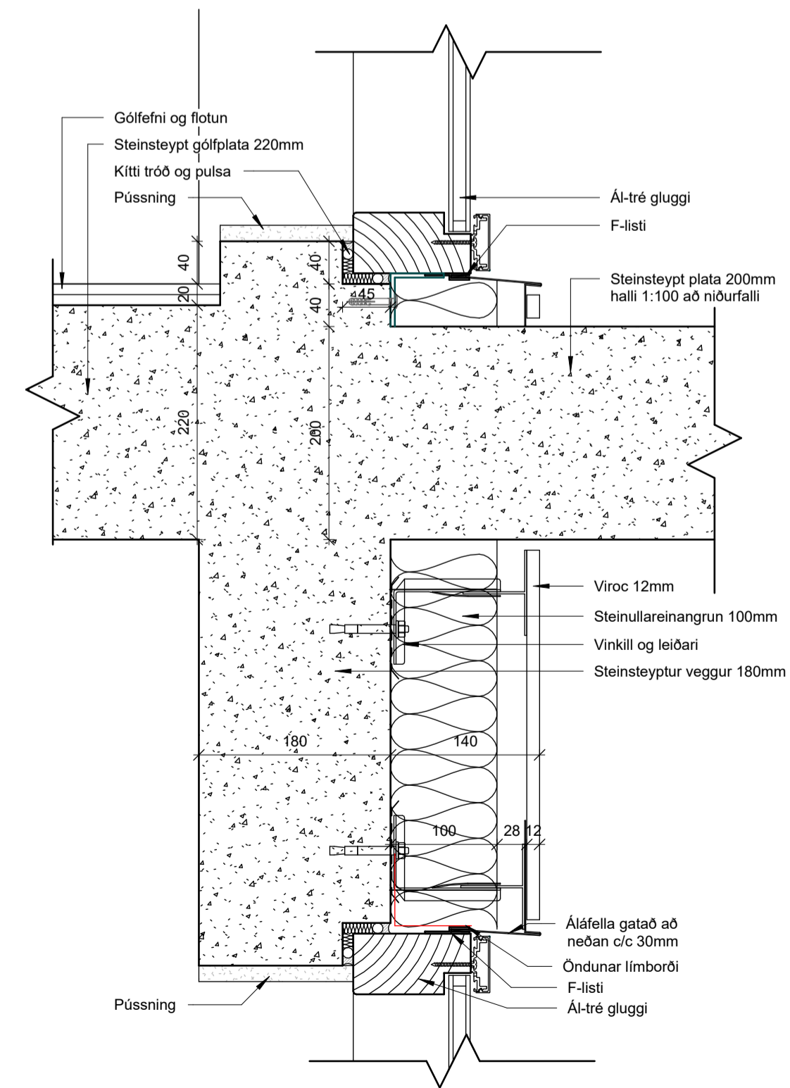
10 Undir gólfsiðan glugga að svölum Viroc 1 : 5
