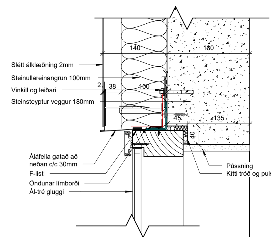
5 Yfir glugga slétt ál 1 : 5
