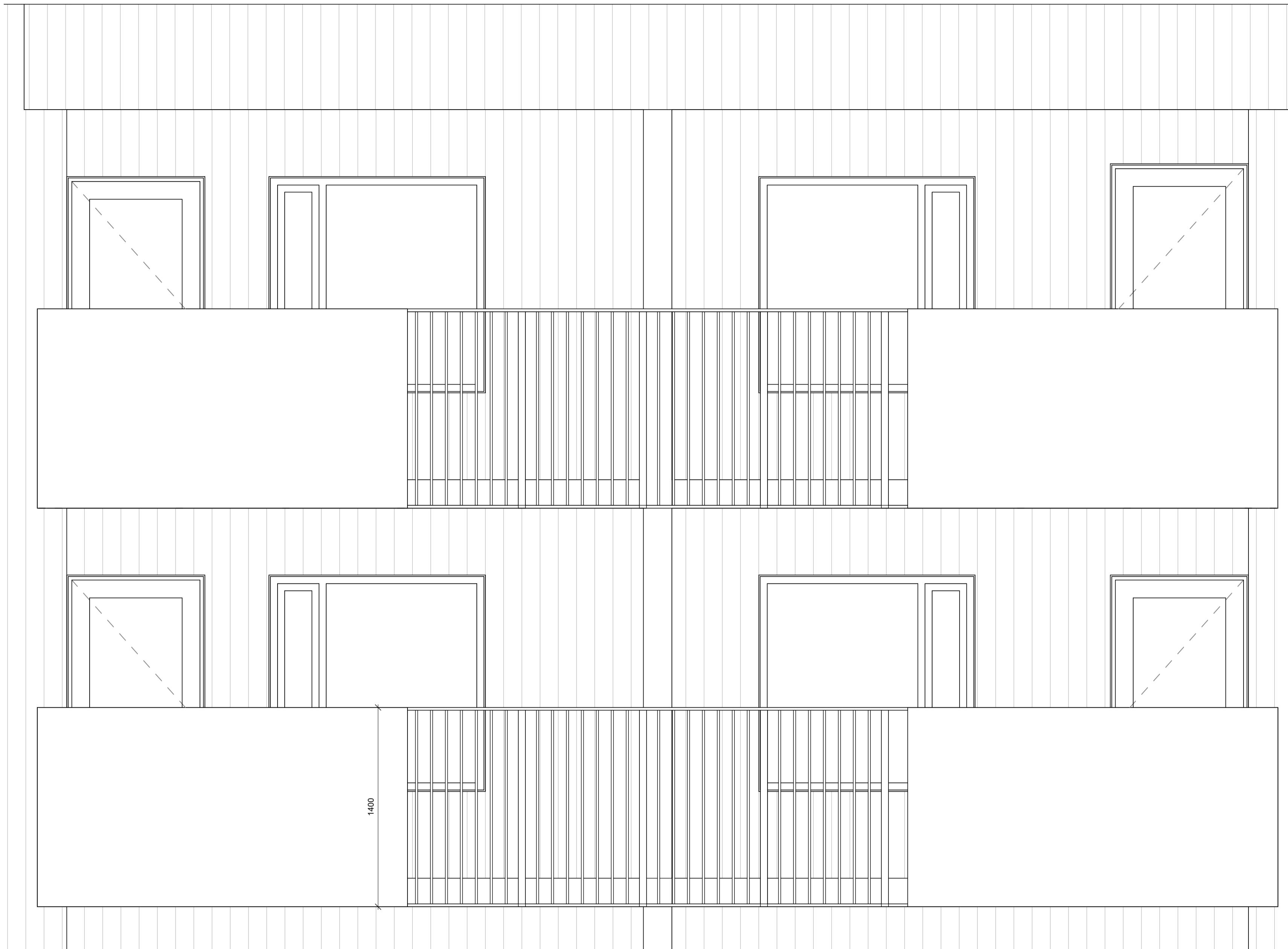
1 Framan við svalir 0205-0206-0306-0307 1 : 20
