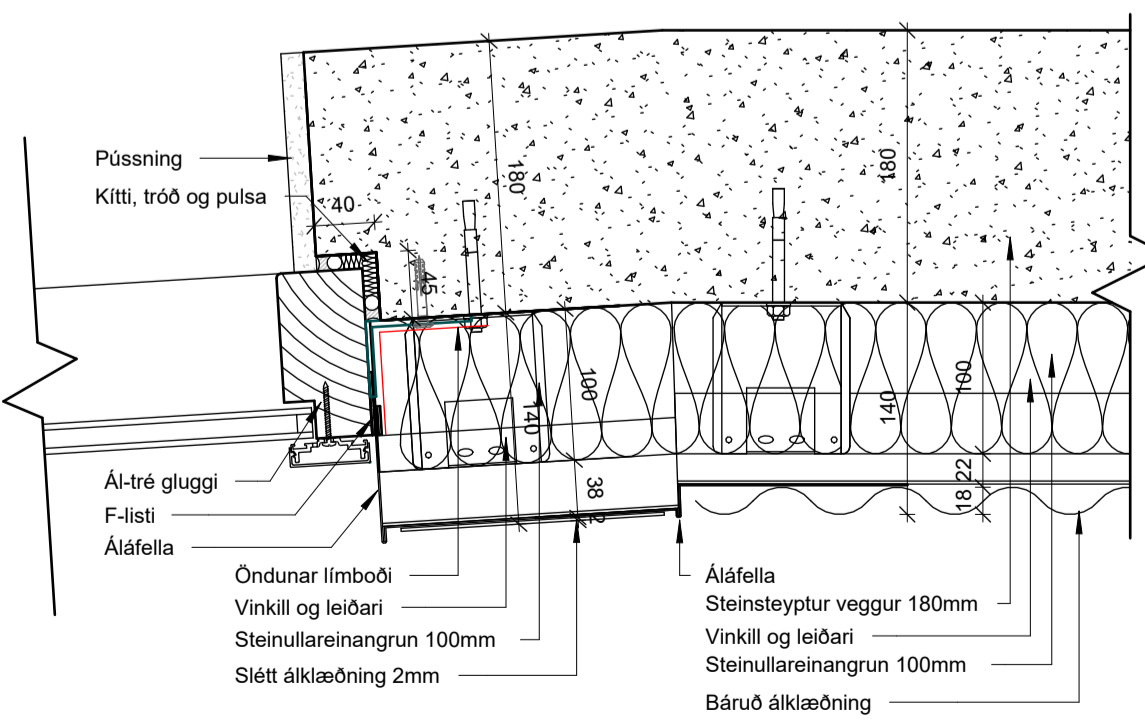
6 Samskeiti slétt að báru 1 : 5
