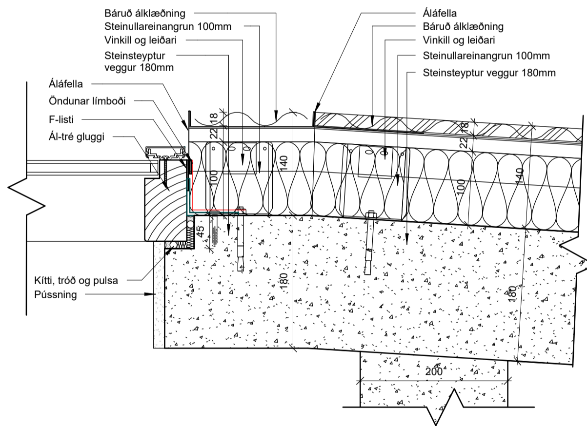
7 Úthorn gleitt báru 1 : 5
