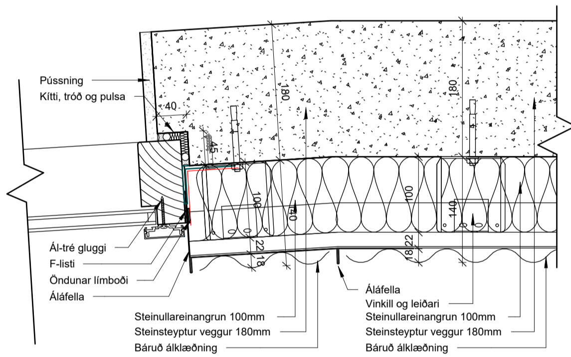
5 Samskeiti báruál 1 : 5
