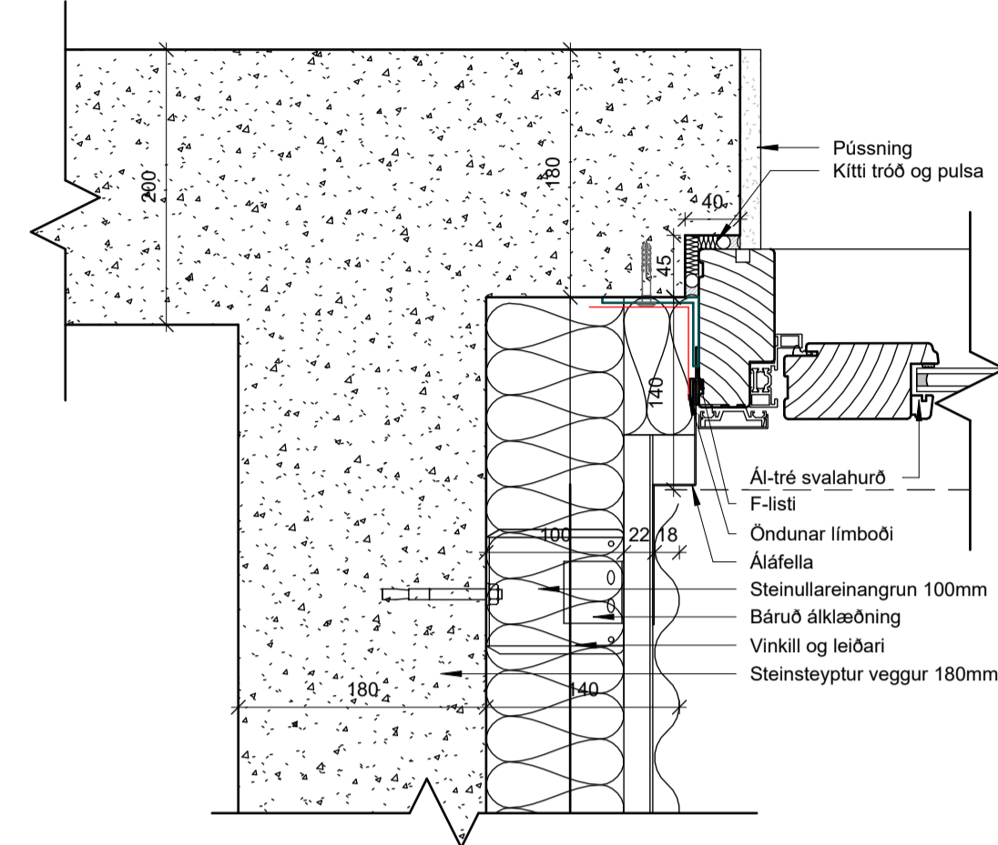
3 Innhorn slétt vs báruál með svalahurð 1 : 5
