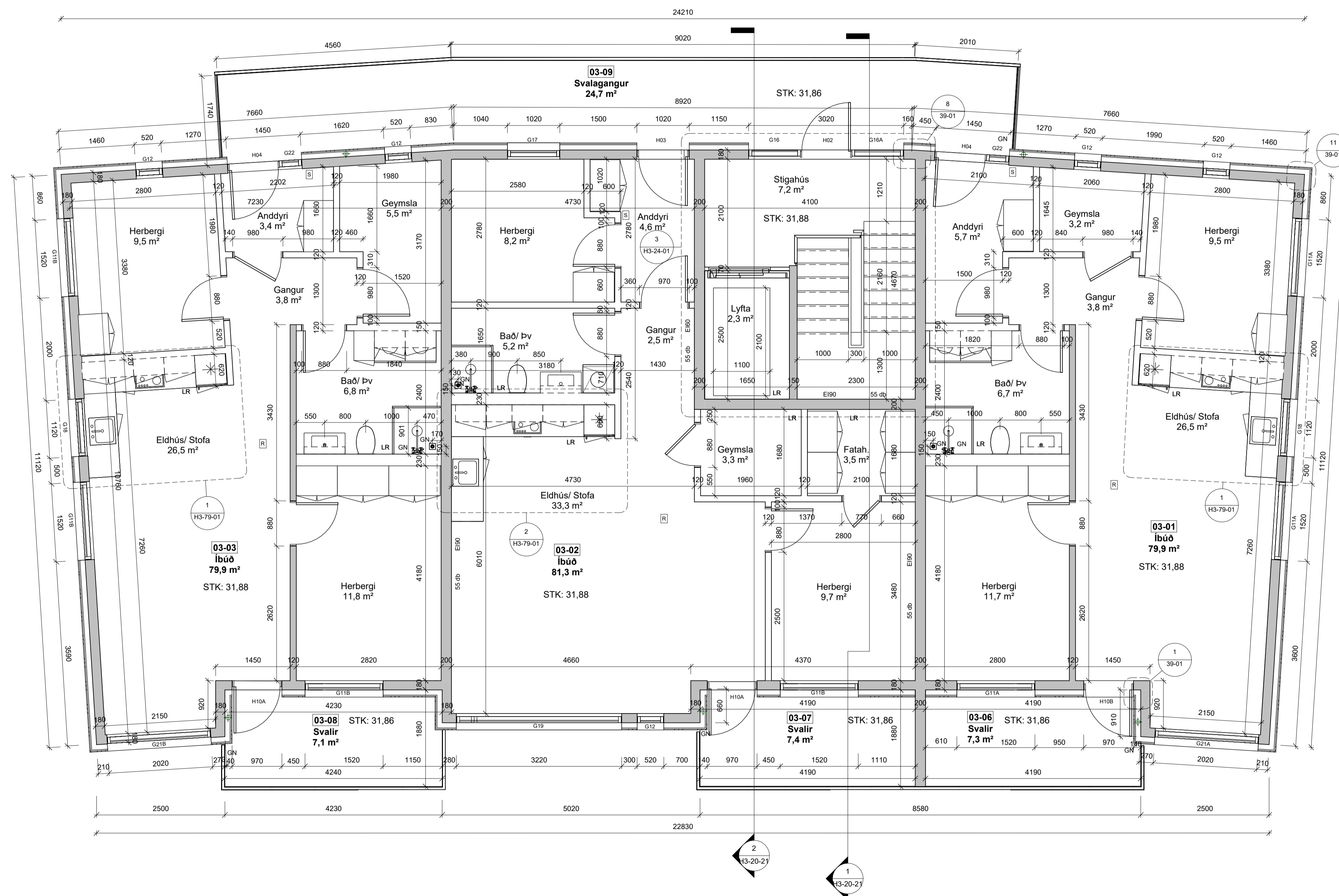
1 3. hæð 1:50
