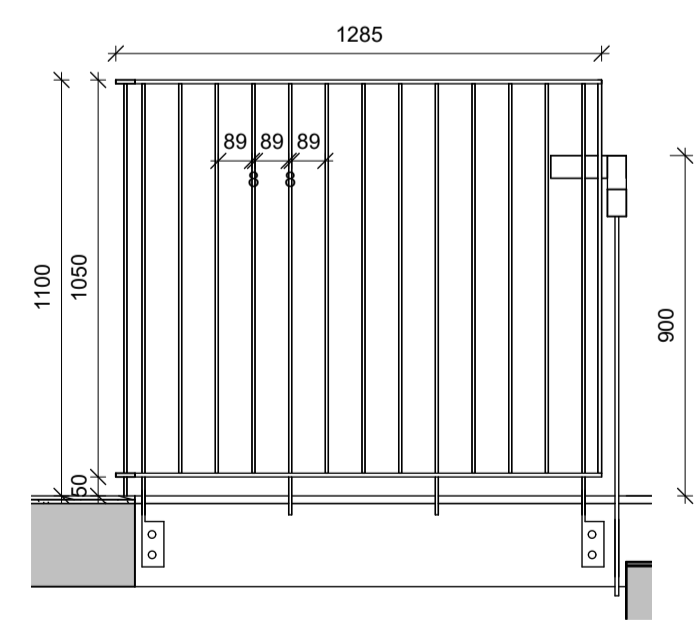
5 Handrið 3. hæð 1:20
