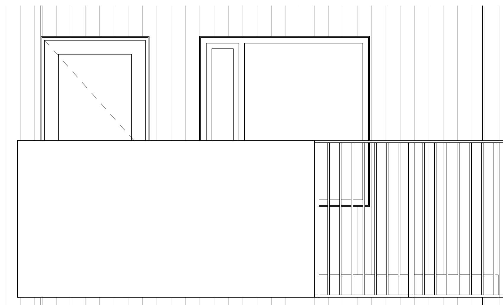
3 H3 - Framan við Svalir 0207-0308 1 : 20
