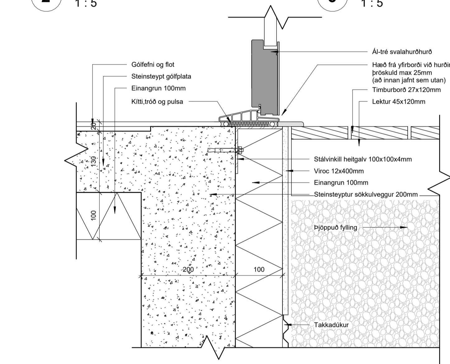
7 Svalahurð að palli 1 : 5
