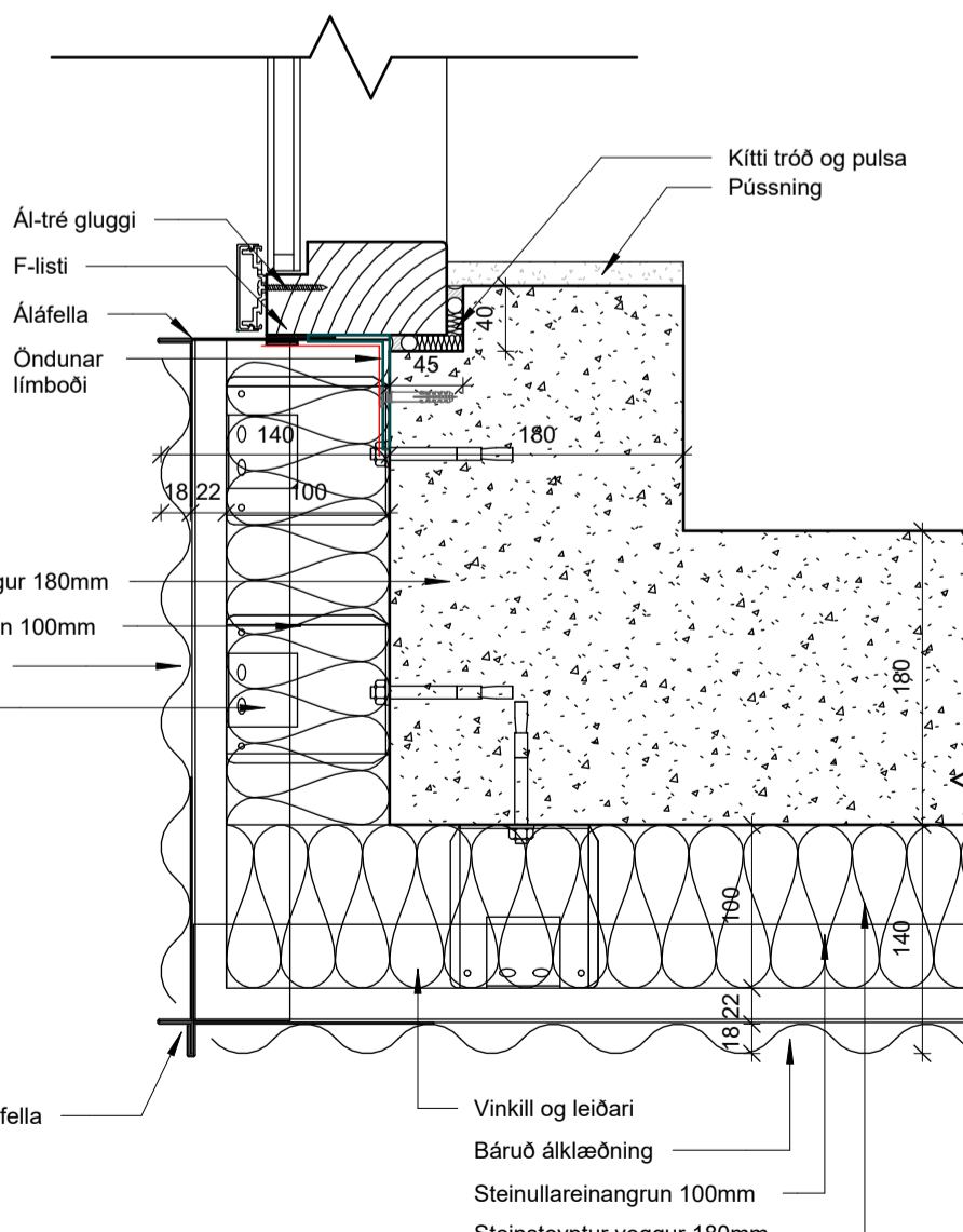
10 Úthorn báruál með glugga 1 : 5
