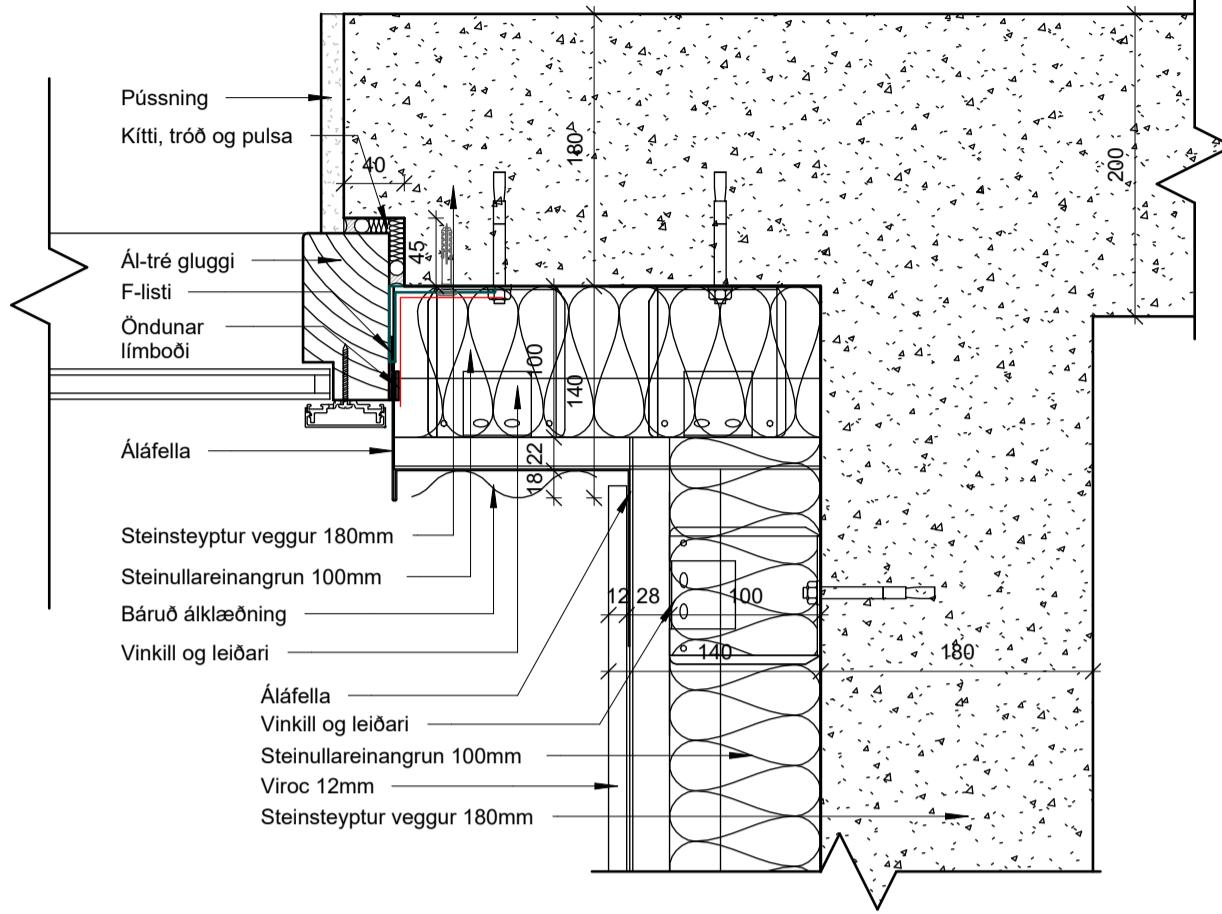
2 Innhorn báruál við Viroc með glugga 1 : 5
